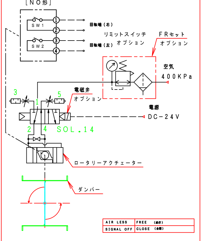
フローシート図 [TA2-0402D-□□-□□□]
